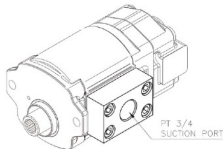
Ansaugflansch ZX75 (AP2D36, AP2D38)
