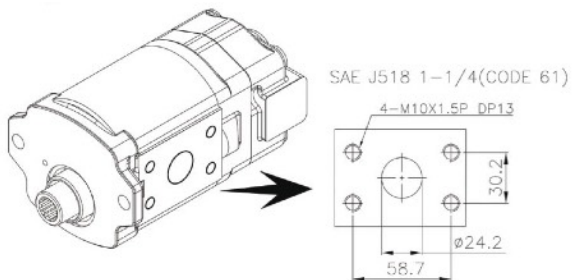
Ansaugflansch ZX60 (AP2D25, AP2D28)
