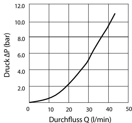
In beide Richtungen vollständig geöffnetes Ventil
